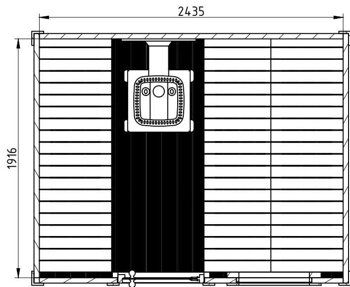
A-A (1:30)
